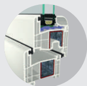
6 kamrás rendszer síkban eltolt szárny
